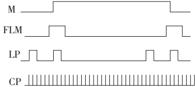
图 3 引脚信号的时序关系 2
