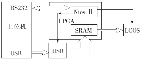
图 1 LCOS 系统原理图
