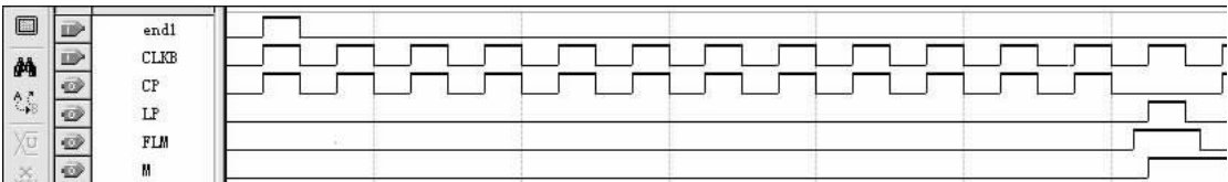
图 4 Nios II 控制器的功能仿真波形 Fig. 4 Function simulation waveshape of LC controller
