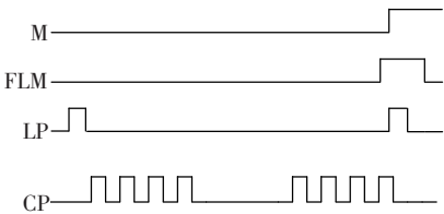
图 2 引脚信号的时序关系 1
